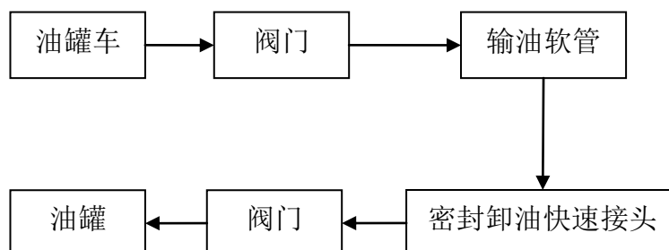
图 2-2 柴油卸油工艺流程示意图
