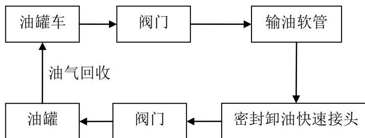
图 2-1 汽油卸油工艺流程示意图
